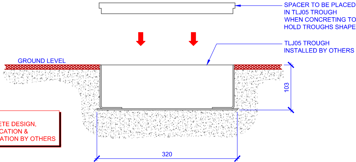
SECTION VIEW TLJ05 TROUGH & SPACER BAR N.T.S.
