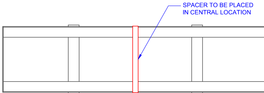
TOP VIEW TLJ05 TROUGH & SPACER BAR N.T.S.
